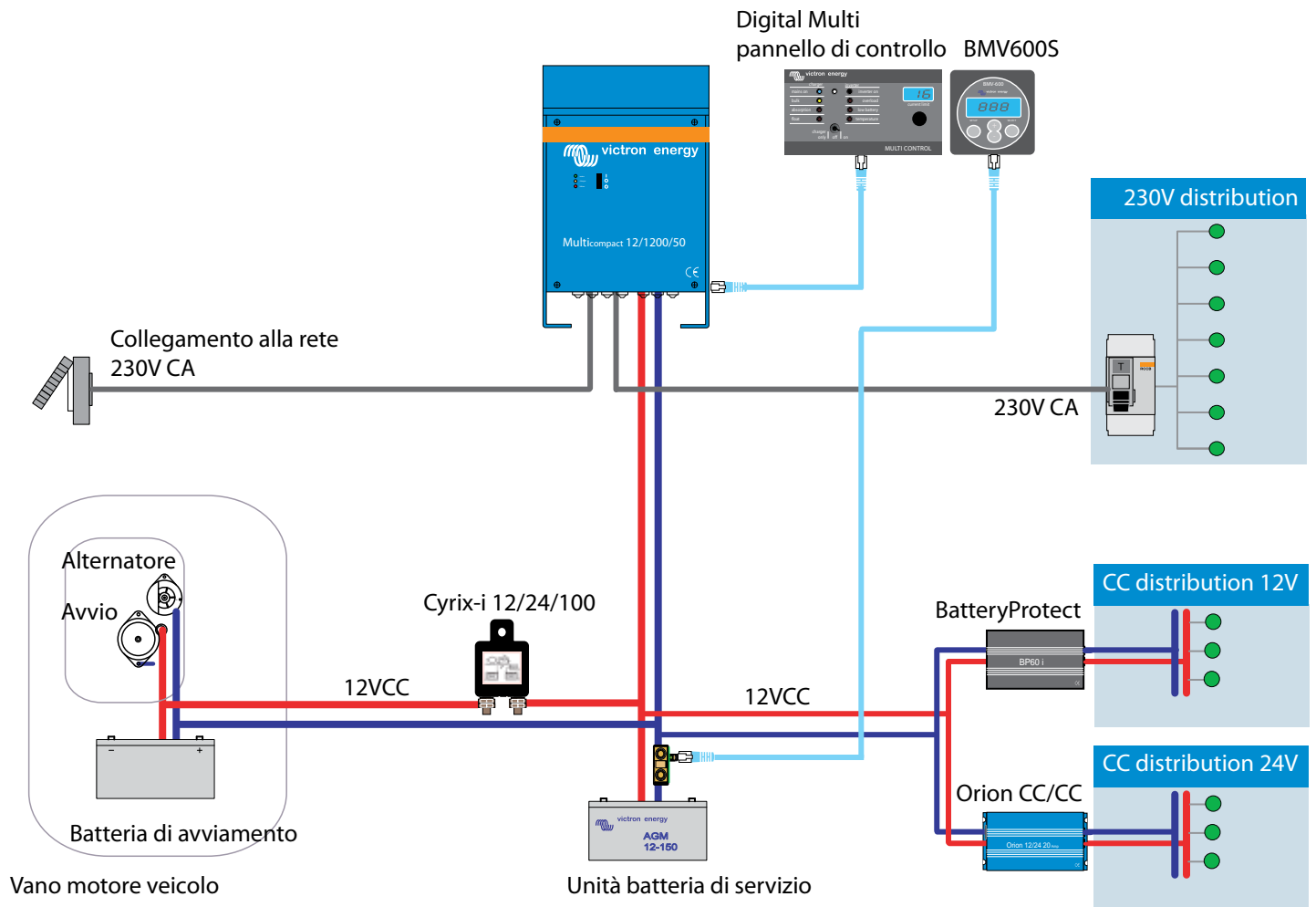
Schema d'insieme dell'impianto nelle ambulanze di Parigi.
