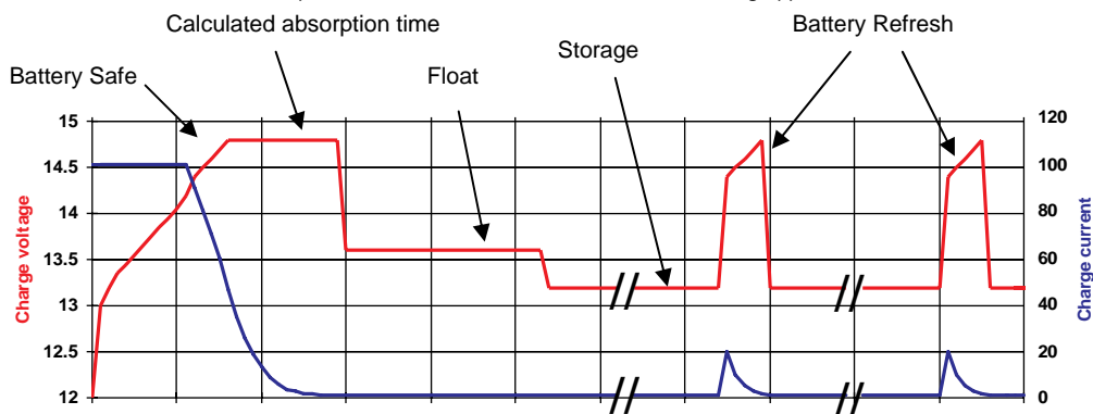
Fig. 4: Curva carica adattiva 4 fasi
