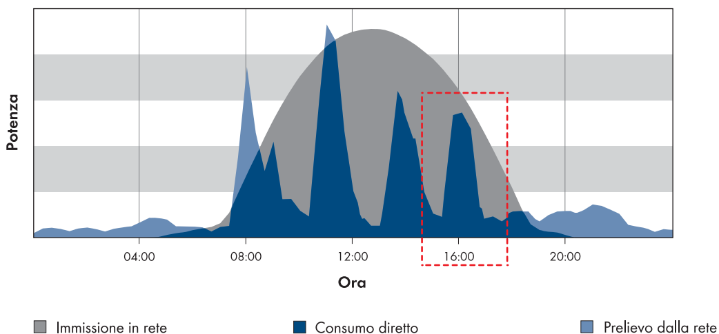
figura 2: Profilo giornaliero di un impianto fotovoltaico, del consumo elettrico e dell'autoconsumo, con controllo dei carichi (esempio) Il riquadro rosso in questo esempio indica lo spostamento del picco di carico al pomeriggio. Grazie al controllo automatico mediante il sistema di gestione energetica, il funzionamento della lavatrice è spostato in una fascia oraria in cui è disponibile energia FV conveniente. In questo modo si aumenta l'autoconsumo di energia FV e si riducono i costi per l'energia prelevata dalla rete.
