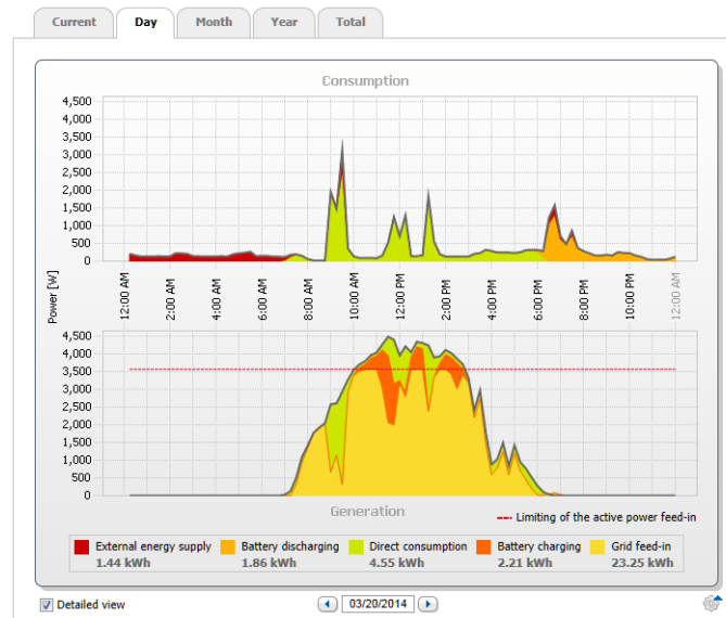
figura 15: Visualizzazione di produzione FV e consumo elettrico su Sunny Portal (esempio 2)
