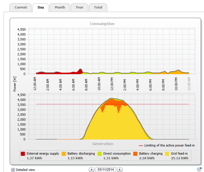
figura 14: Visualizzazione di produzione FV e consumo elettrico su Sunny Portal (esempio 1)
