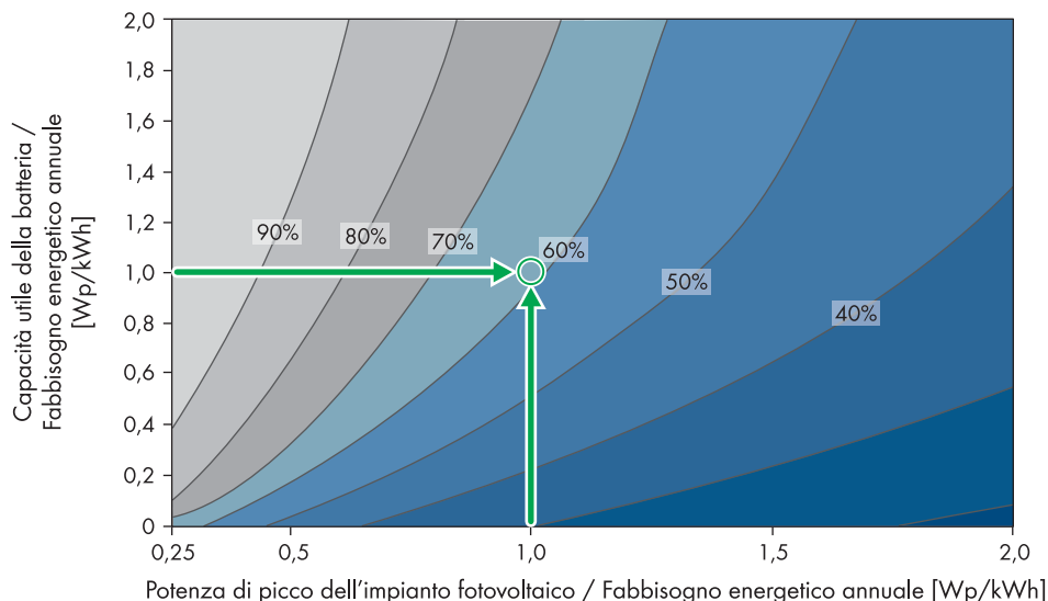
figura 28: Stima della quota di autoconsumo con accumulo temporaneo
