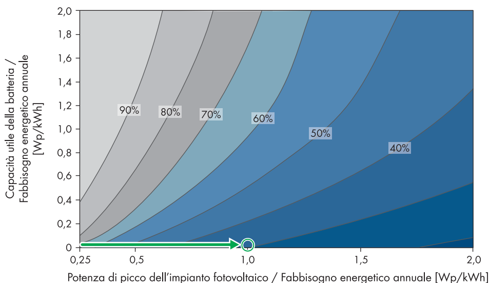
figura 27: Stima della quota di autoconsumo senza accumulo temporaneo
