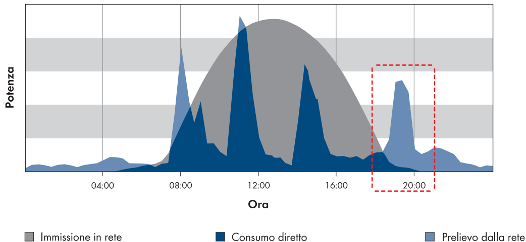
figura 1: Profilo giornaliero di un impianto fotovoltaico, del consumo elettrico e dell'autoconsumo, senza controllo dei carichi (esempio) Il riquadro rosso in questo esempio indica un picco di carico alla sera. Quest'ultimo è dovuto ad es. a una lavatrice che viene attivata manualmente la sera.
