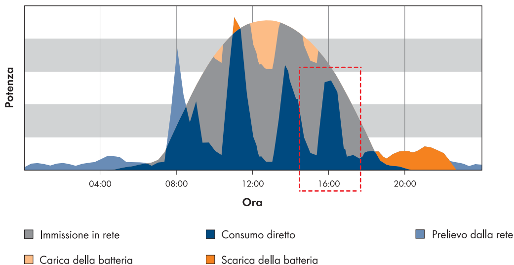
figura 5: Profilo giornaliero di un impianto fotovoltaico, del consumo elettrico e dell'autoconsumo, con controllo dei carichi e accumulo temporaneo (esempio di SMA Integrated Storage System)
