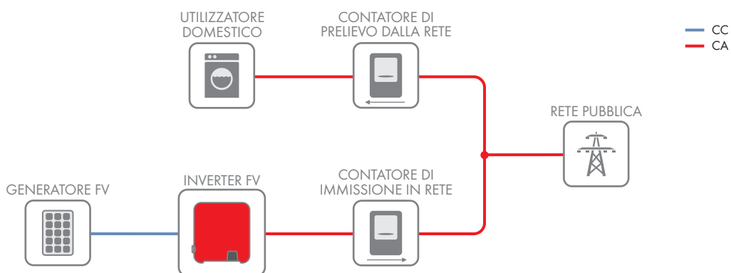
figura 12: Installazione dei contatori in un impianto di immissione (esempio)
