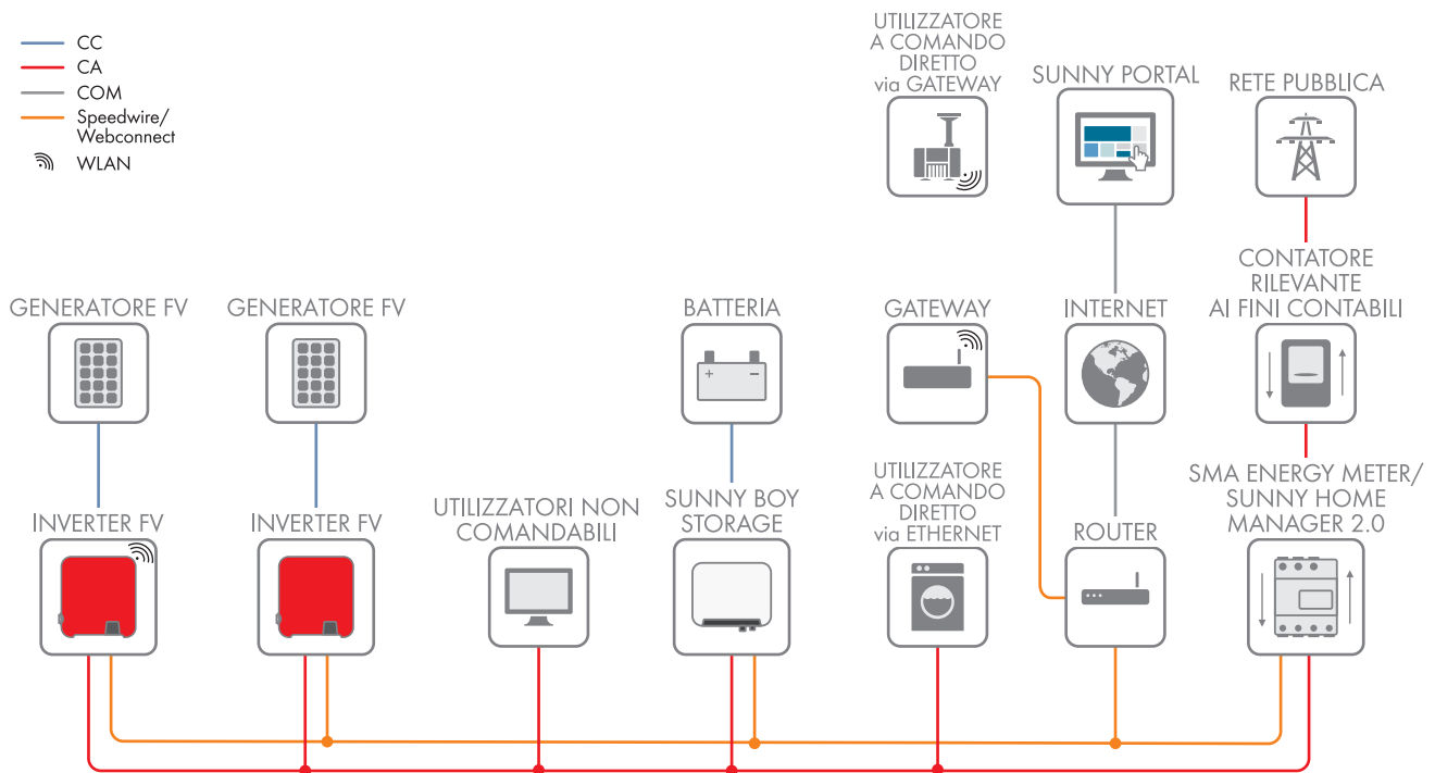
figura 3: Impianto fotovoltaico con Sunny Home Manager (esempio)
