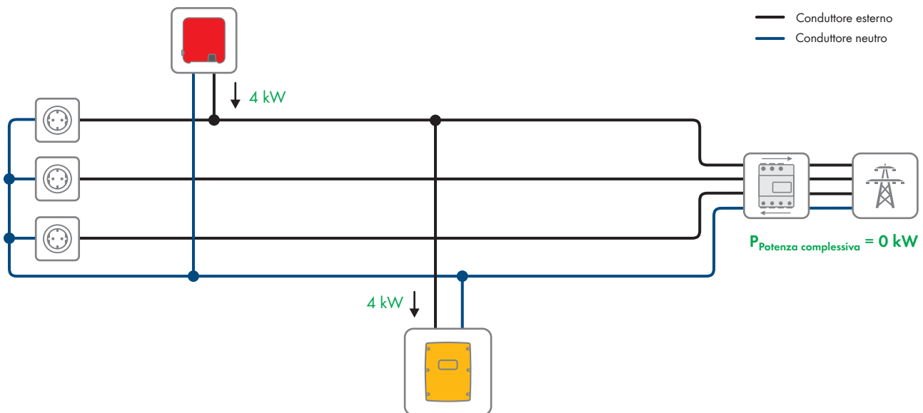
figura 19: L'inverter con batteria carica la batteria.
