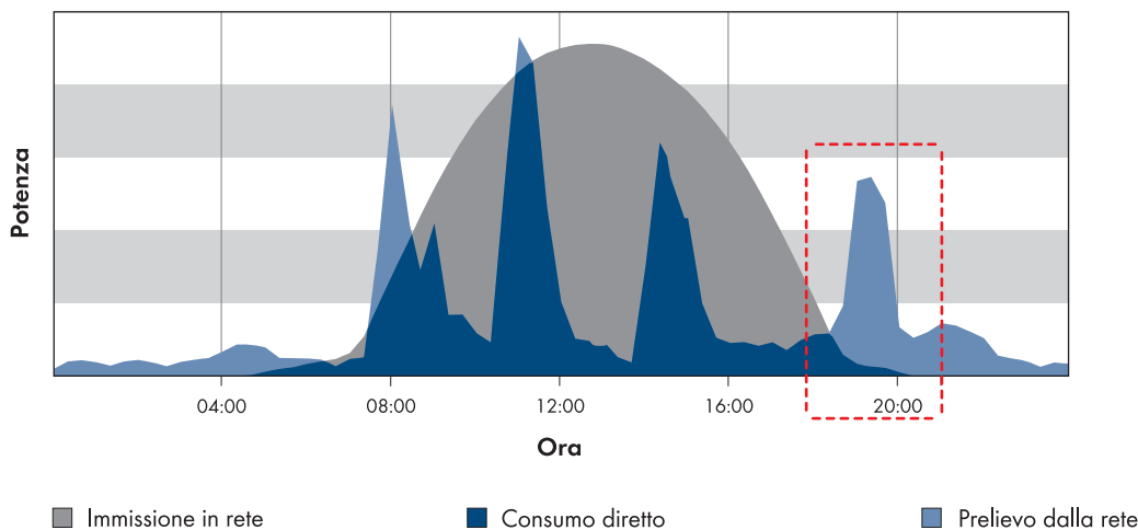
figura 4: Profilo giornaliero di un impianto fotovoltaico, del consumo elettrico e dell'autoconsumo, senza controllo dei carichi né accumulo temporaneo (esempio)
