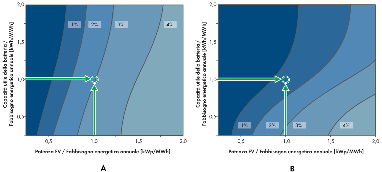
figura 18: Perdite annuali in percentuale riferite alla produzione FV con limitazione dell'immissione al 60%, con (A) e senza (B) caricamento della batteria programmato in base alle previsioni
