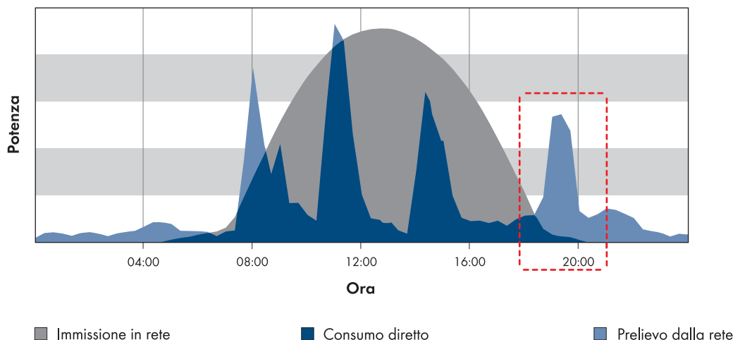
figura 7: Profilo giornaliero di un impianto fotovoltaico, del consumo elettrico e dell'autoconsumo, senza controllo dei carichi né accumulo temporaneo (esempio)
