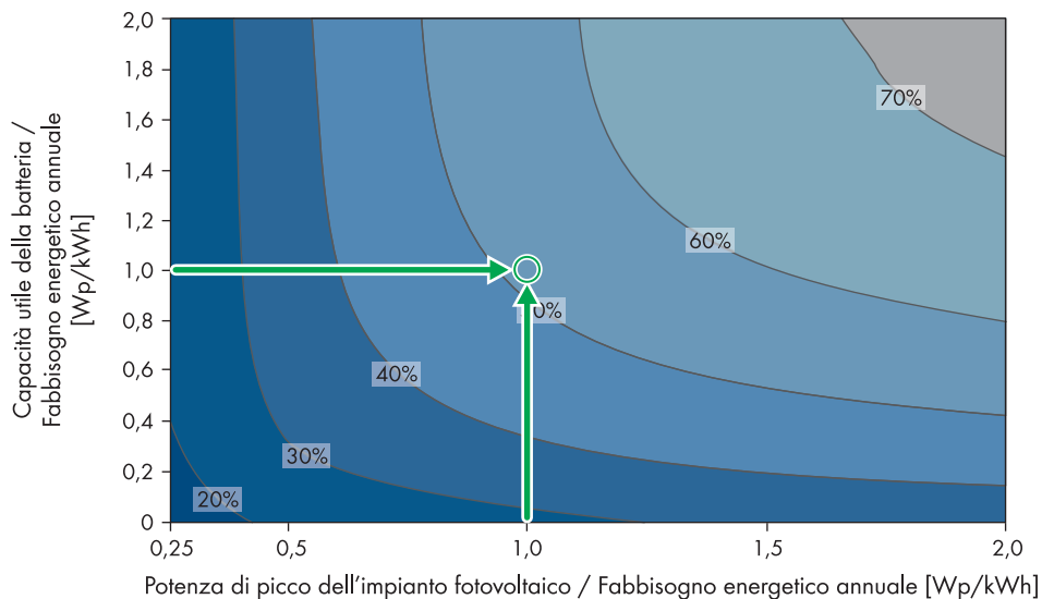
figura 30: Stima della quota di autarchia con accumulo temporaneo
