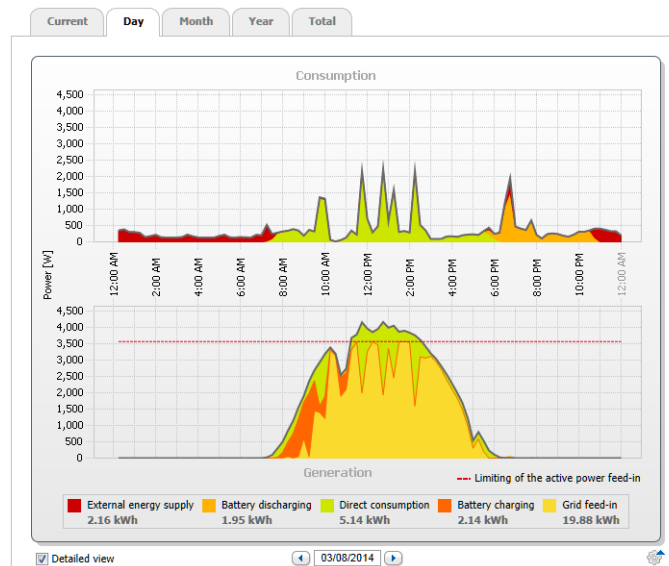
figura 16: Visualizzazione di produzione FV e consumo elettrico su Sunny Portal (esempio 3)
