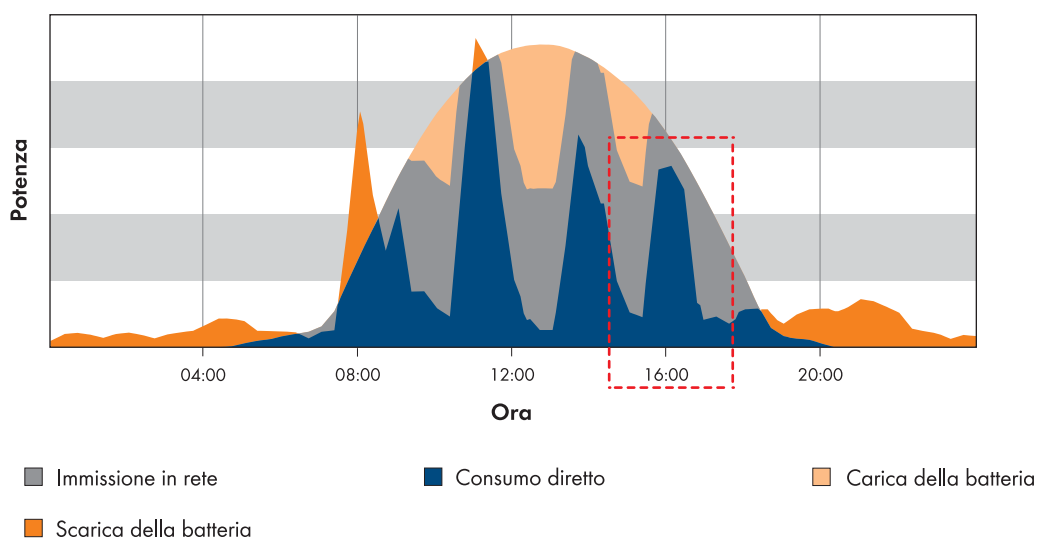
figura 8: Profilo giornaliero di un impianto fotovoltaico, del consumo elettrico e dell'autoconsumo, con controllo dei carichi e accumulo temporaneo (esempio di SMA Flexible Storage System)
