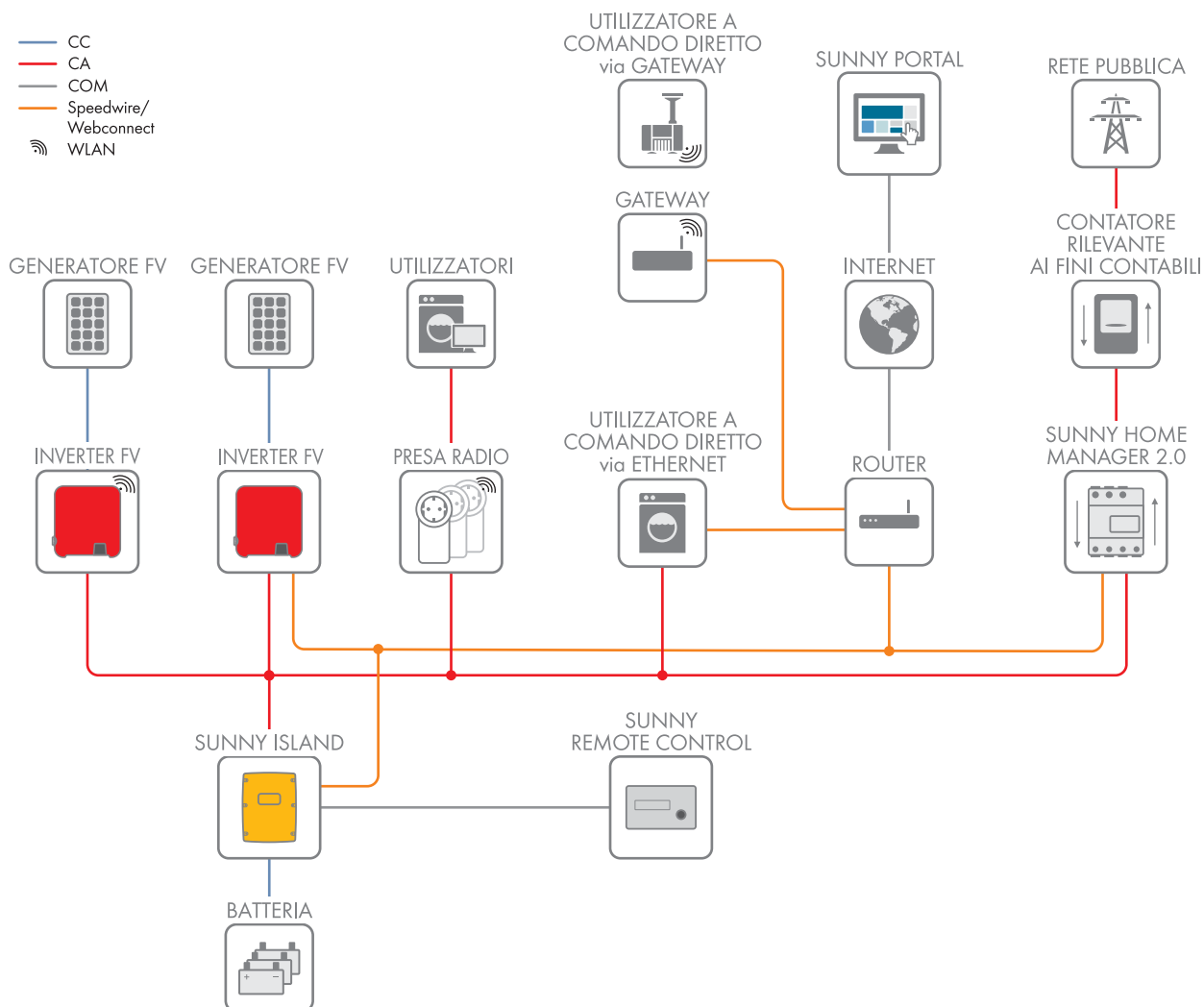
figura 9: Impianto FV con SMA Flexible Storage System con Sunny Island (esempio)
