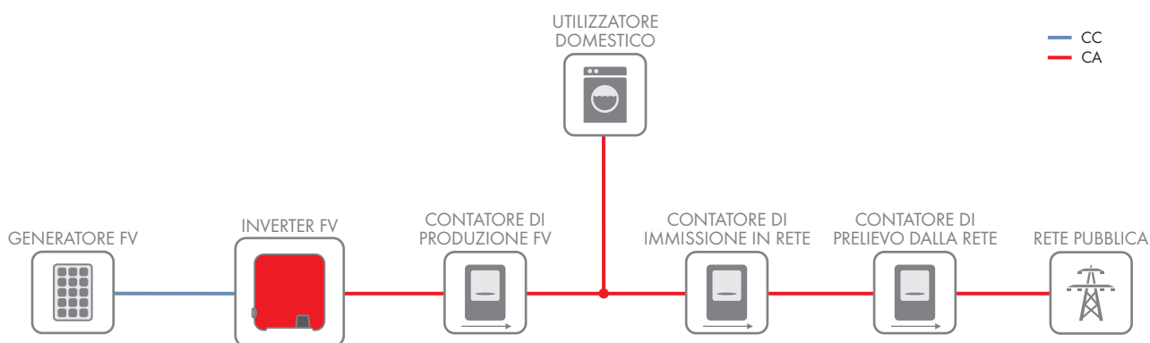
figura 11: Installazione dei contatori in un impianto per autoconsumo (esempio)
