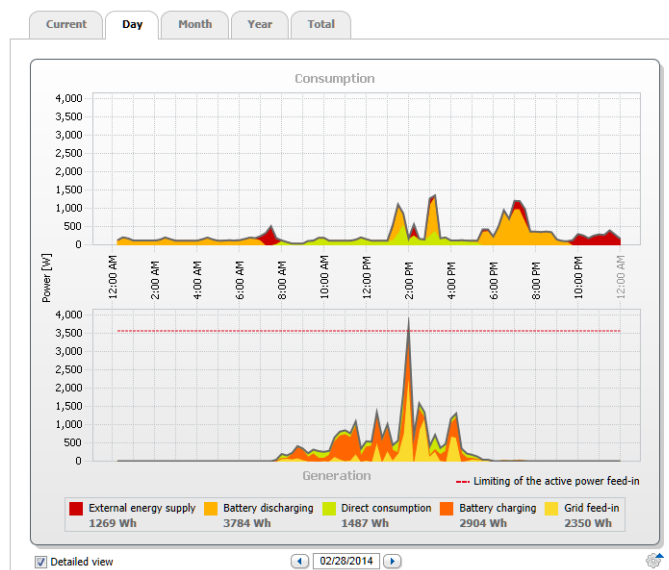
figura 17: Visualizzazione di produzione FV e consumo elettrico su Sunny Portal (esempio 4)
