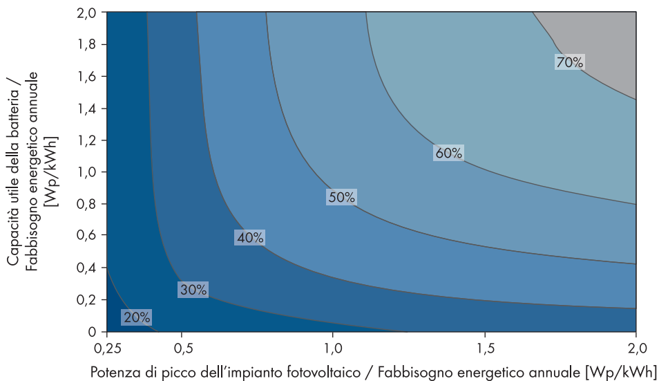
figura 26: Stima della quota di autarchia
