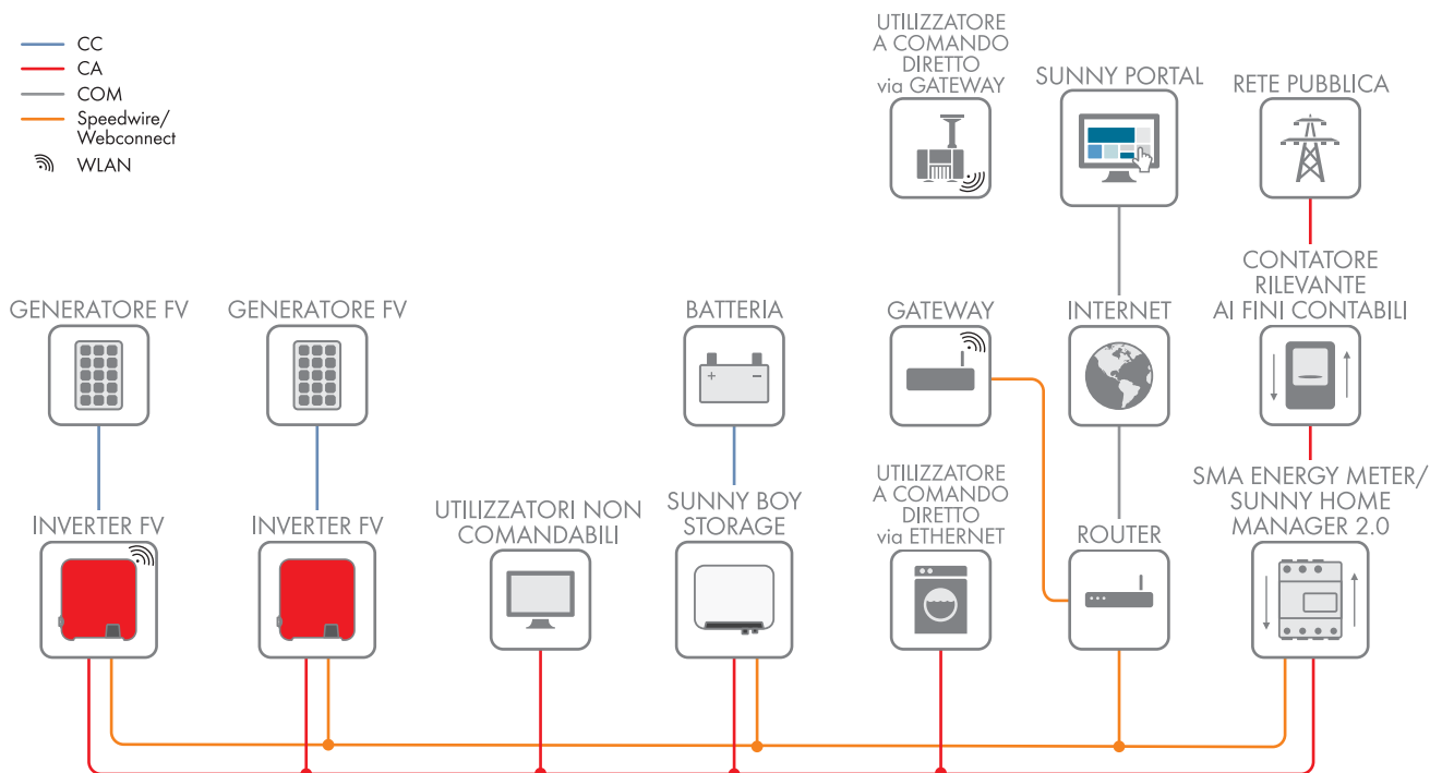
figura 10: Impianto FV con SMA Flexible Storage System con Sunny Boy Storage (esempio)
