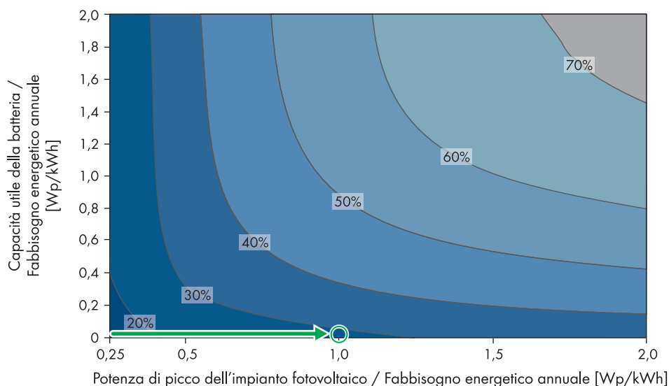
figura 29: Stima della quota di autarchia senza accumulo temporaneo
