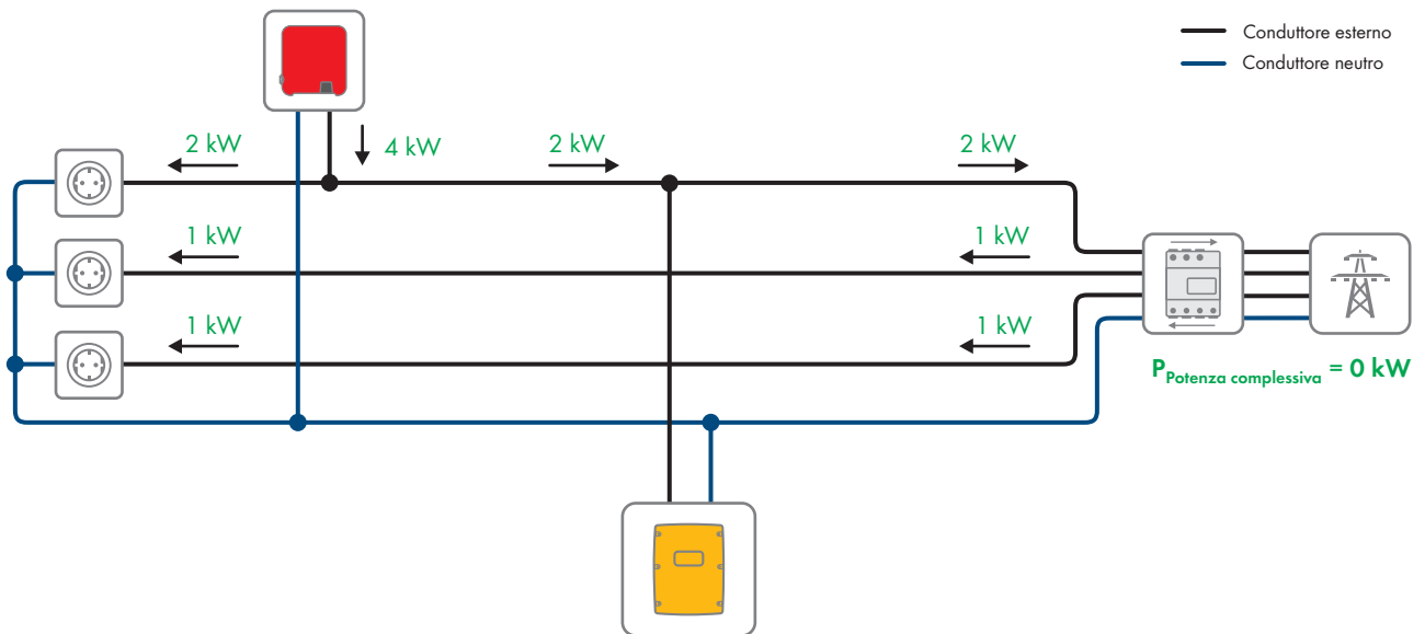
figura 20: Gli utilizzatori elettrici utilizzano tutta la potenza FV.
