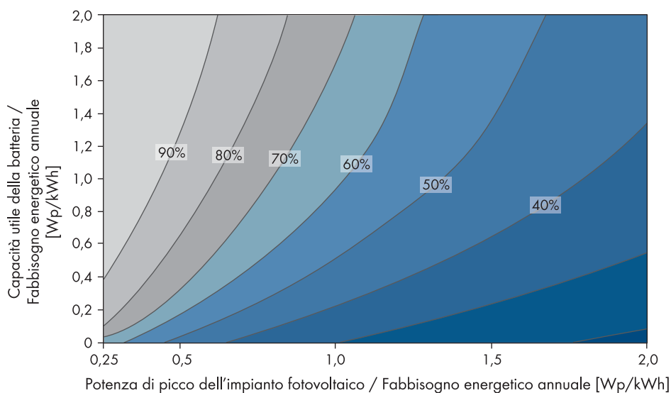
figura 25: Stima della quota di autoconsumo
