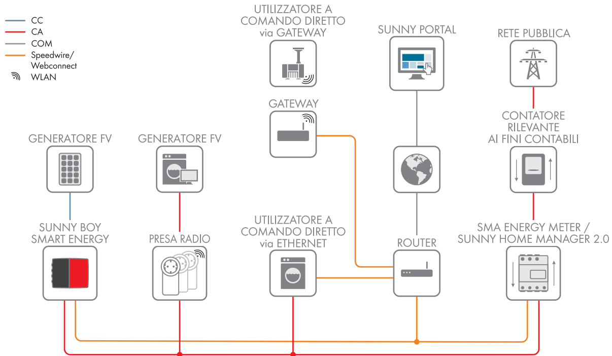
figura 6: Panoramica di SMA Integrated Storage System (esempio)
