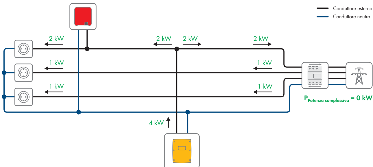
figura 21: L'inverter con batteria alimenta gli utilizzatori con l'energia accumulata.
