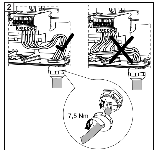
Fronius Symo
