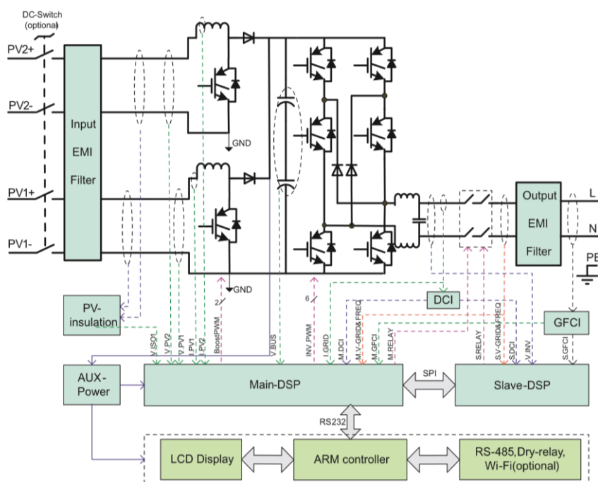
Figura 2-4 Scema elettrico a blocchi
