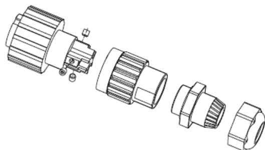
Figura 4-11 connettore di uscita AC
