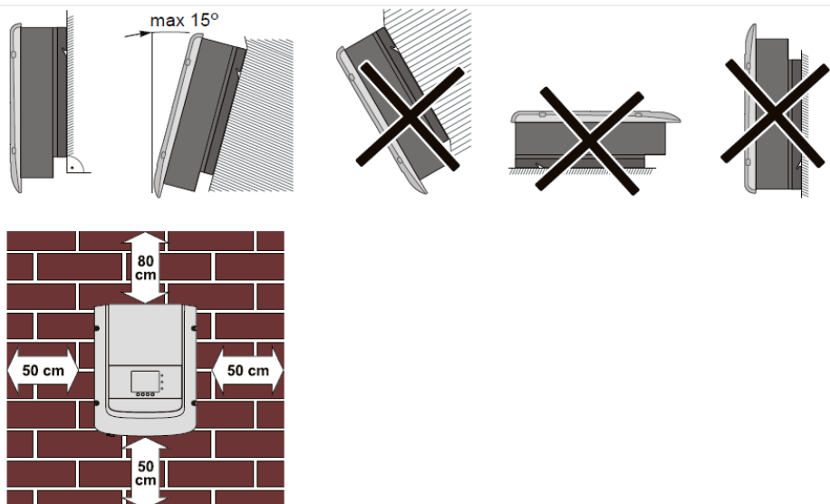
Distanze minime di rispetto per installazione sigola
