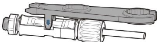
Figura 4-8 Rimozione di un connettore di ingresso DC
