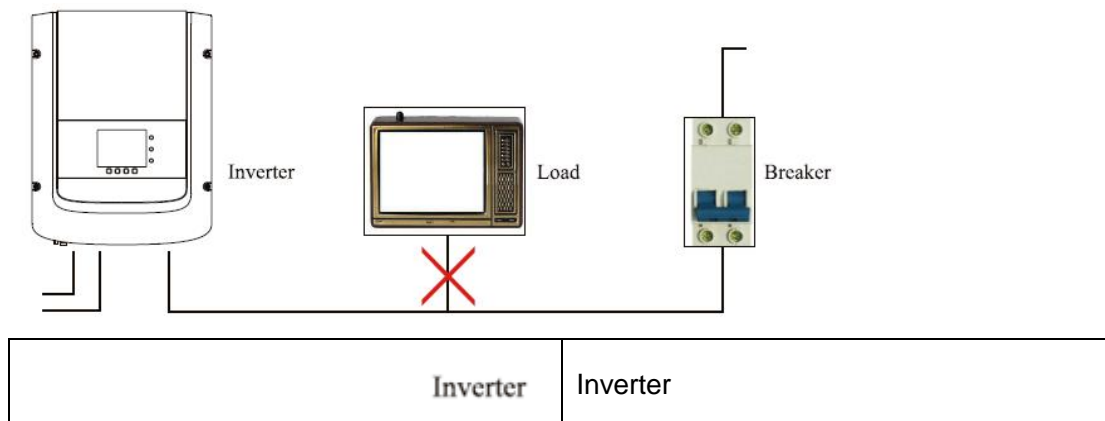
Figura 4-9 NON consentito collegare carichi tra inverter e interruttore
