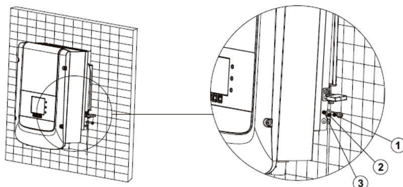
Figura 4-4 Messa a terra
