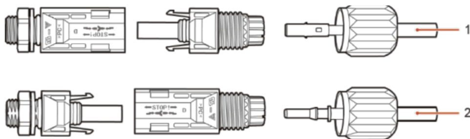
Figura 4-6 Collegamento alimentazione di ingresso DC
