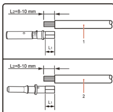
Figura 4-5 Collegamento alimentazione di ingresso DC
