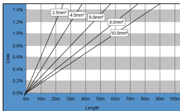
Figura 4-10 lunghezza, sezione e perdite nel conduttore
