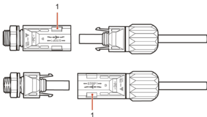
Figura 4-7 Collegamento alimentazione di ingresso DC
