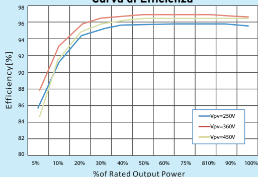
Curva di Efficienza
